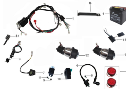
电器组件
