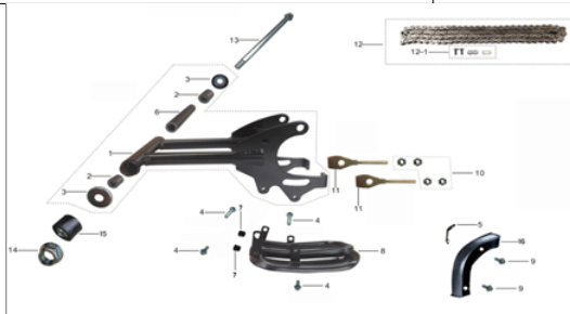
后平叉总成
