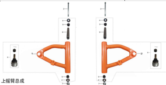
上摇臂总成
