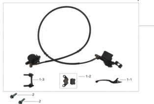
后制动总成
