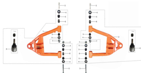
下摇臂总成
