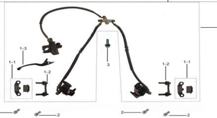
前制动总成
