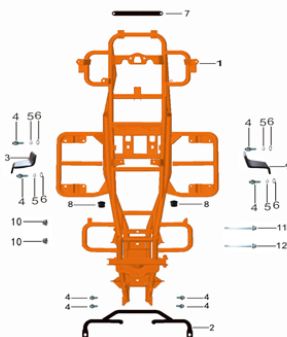
车架总成
