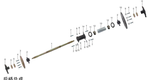
后桥总成
