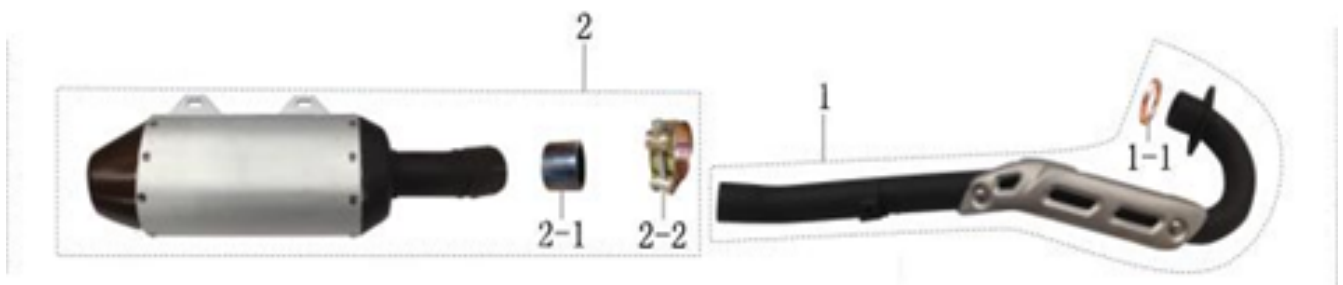
消音器总成
