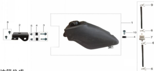
油箱总成
